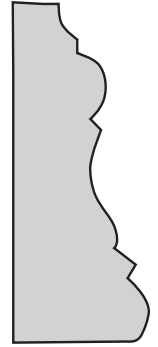
18x45 kehys 049
